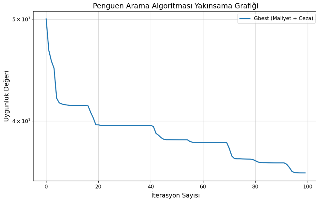
Şekil 2: Penguen Arama Algoritması Yakınsama Grafiği
